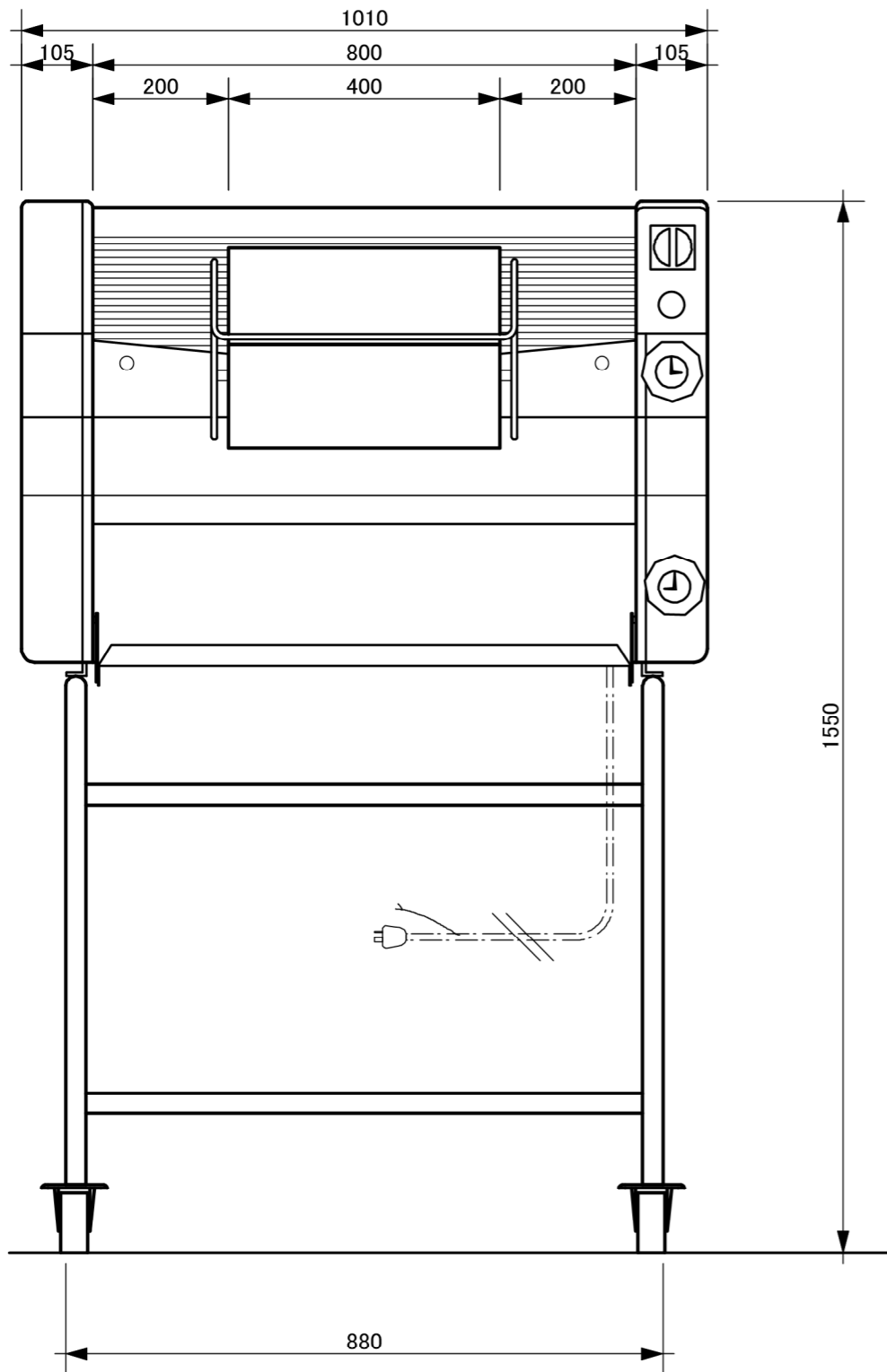
正面図
