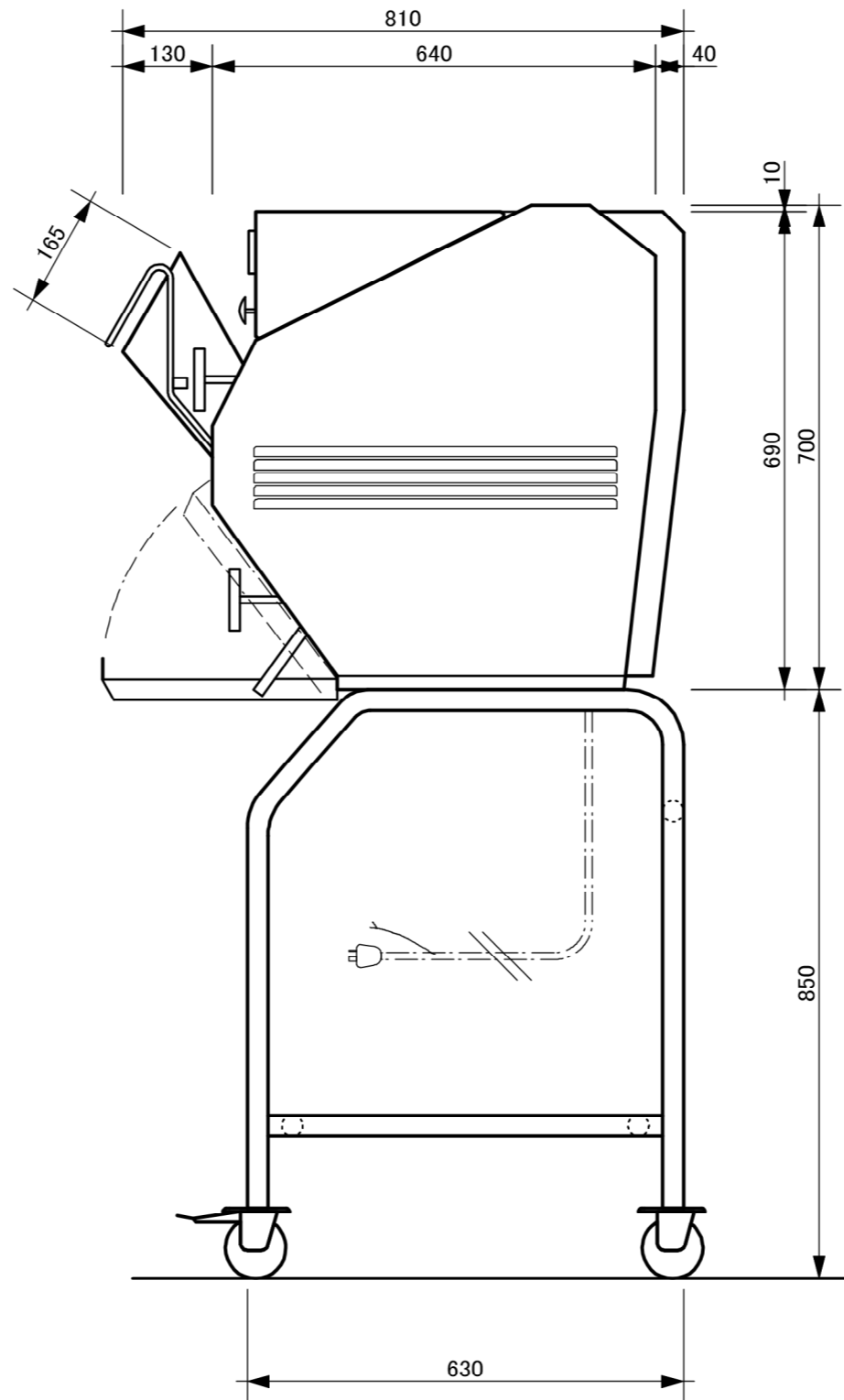
側面図
