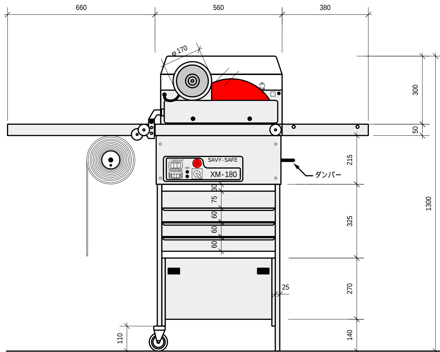
正面図
