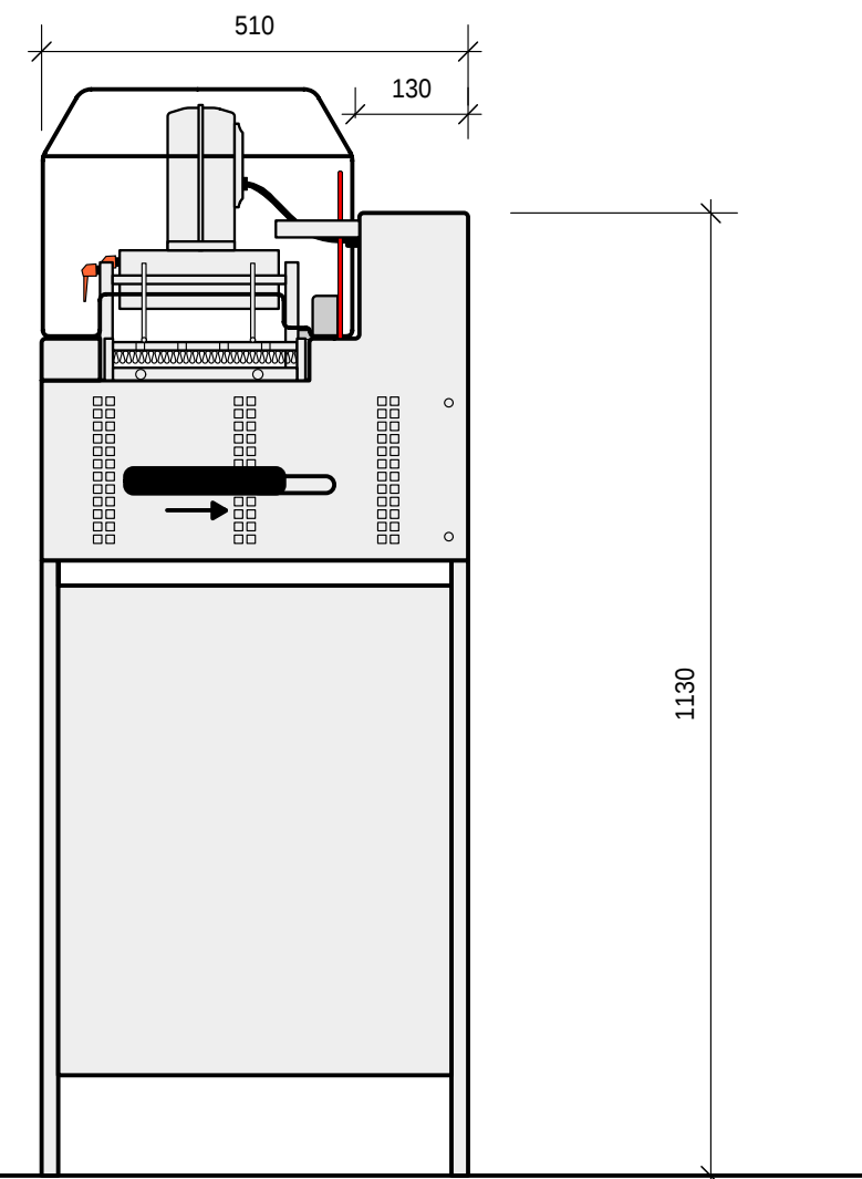
側面図
