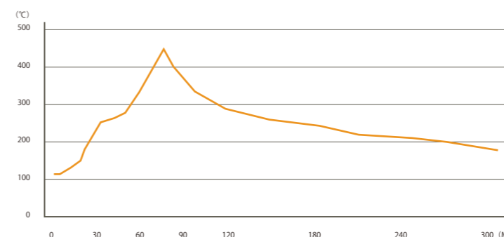
庫内温度(平均)の推移グラフ
